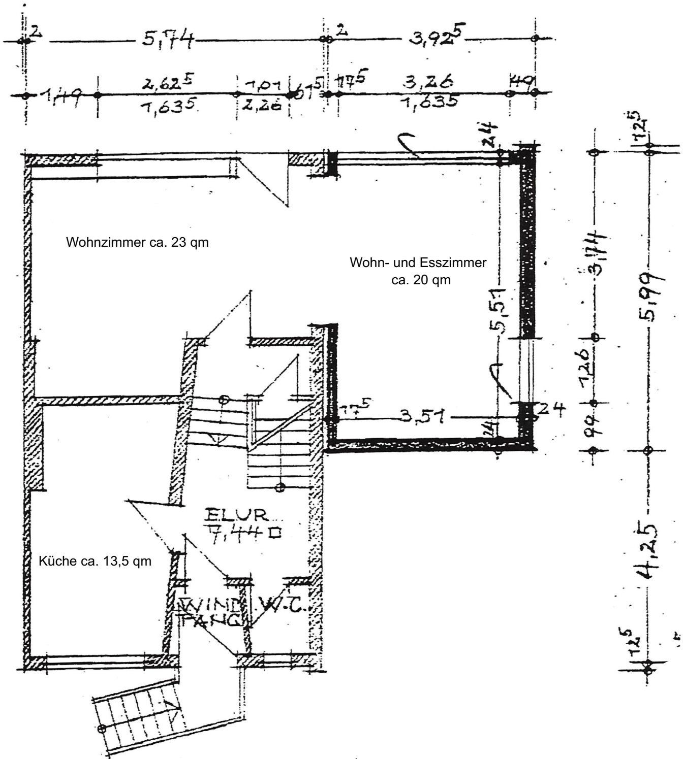
ERDGESCHOSSGRUNDRISS M 1 : 700
